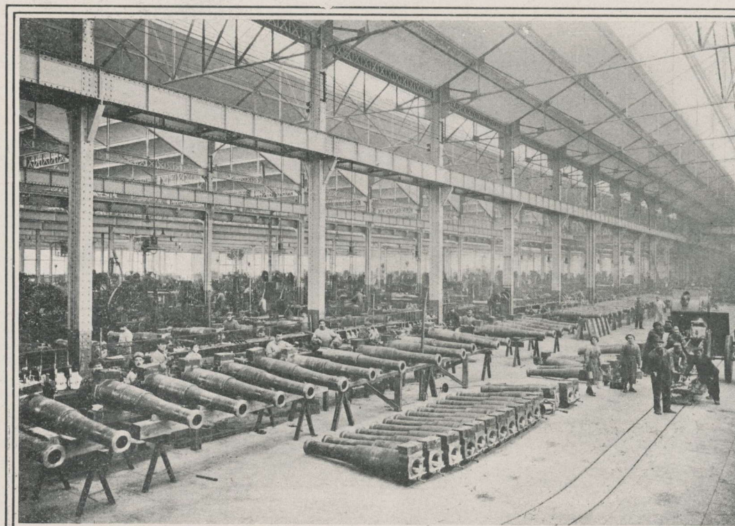
Un des ateliers de la Société d'Outillage Mécanique et d'Usinage d'Artillerie.
