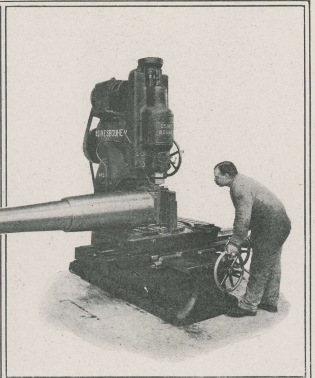
Usinage d'un obusier de 155 sur fraiseuse.
